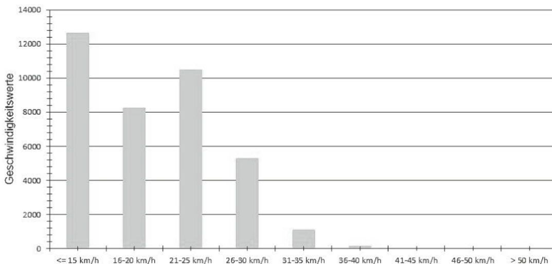
Verteilung Geschwindigkeit
