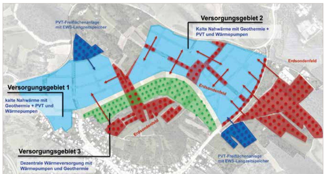
Im Bild: Schematische Darstellung einer möglichen Energieversorgungsvariante für den Hafner – bei der exakten Abgrenzung der Energieerzeugungsf lächen im weiteren Planungsprozess wird der Erhalt vorhandener Biotope und hochwertiger Freiflächen von besonderer Bedeutung sein.
